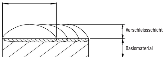
Schweissraupe, überlappend, 4-12mm
